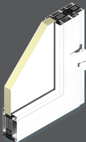
Innenansicht Glasfalz mit Standard-Aufsatztürbändern
