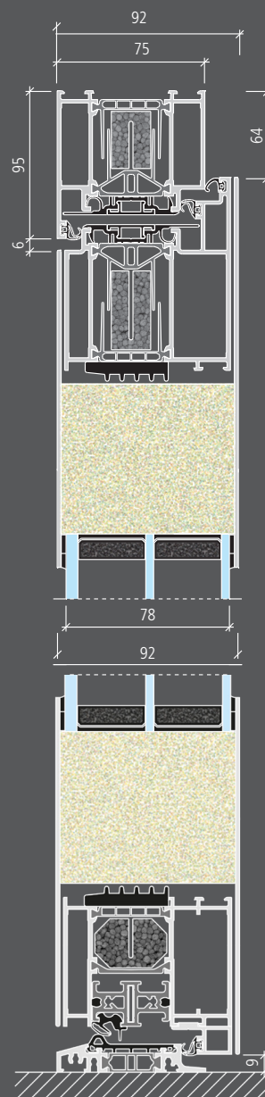
KÖSTER ADVANCE 88 mit einem 95 mm Blendrahmen
