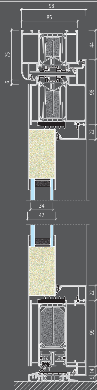
Ausführung mit rundem Blendrahmen (optional): KÖSTER ADVANCE 98
