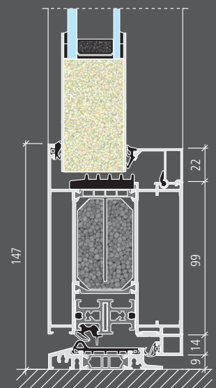
Ausführung mit rundem Blendrahmen (optional): KÖSTER ADVANCE 98
