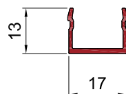
Gewebeprofil 17x13 mm TN 456520
